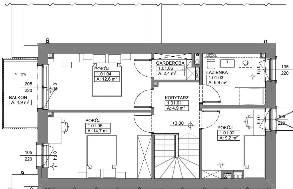
KONDYGNACJA 2
